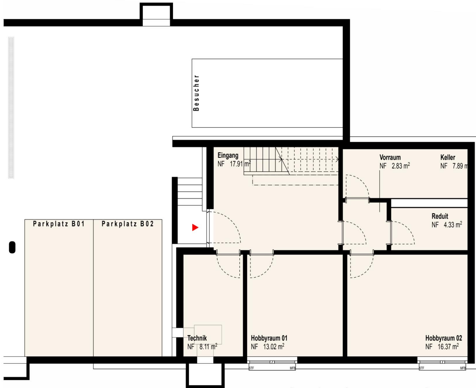
Untergeschoss Haus B
